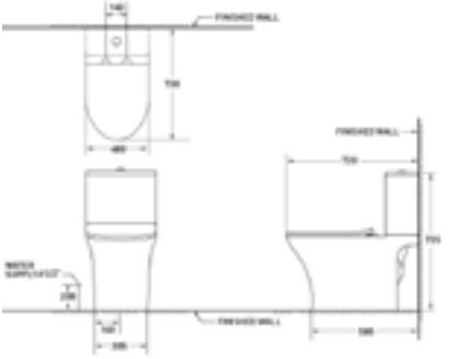
AQ 905789/9179 2 INCH PIPE PE สุขภัณฑ์สองชั้น ขนาด 400 x 720 x 735 มม. + แวกซ์กันซึม/ชุดน็อตยึด + ปริมาณน้ำ/ปุ่มฟลัช: 3/6 ลิตร + ระบบฟลัช: SIPHON JET + ขนาดท่อน้ำ: 2 นิ้ว + ฝารองนั่ง: PE + ฝาเปิด-ปิด แบบ SOFT CLOSED แบบปุ่มกดตลอดได้ + ระยะท่อน้ำจากกำแพงคกแล้ว 30 ซม. 2,690บาท
